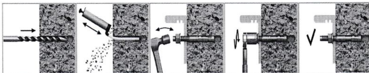
Рис. 3. Порядок установки механических анкеров
